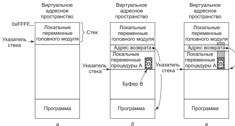
Рис. 9.19. Складывающиеся ситуации: a — при работе основной программы; б — после вызова процедуры A ; в — при переполнении буфера, показанного серым цветом
