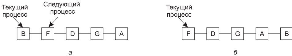
Рис. 2.22. Циклическое планирование: а — список процессов, находящихся в состоянии готовности; б — тот же список после того, как процесс В исчерпал свой квант времени
