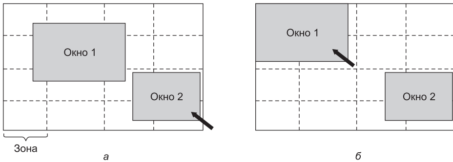
Рис. 5.32. Использование зон подсветки экрана: а — при выборе окна 2 оно не перемещается; б — при выборе окна 1 оно перемещается, чтобы уменьшить количество подсвечиваемых зон
