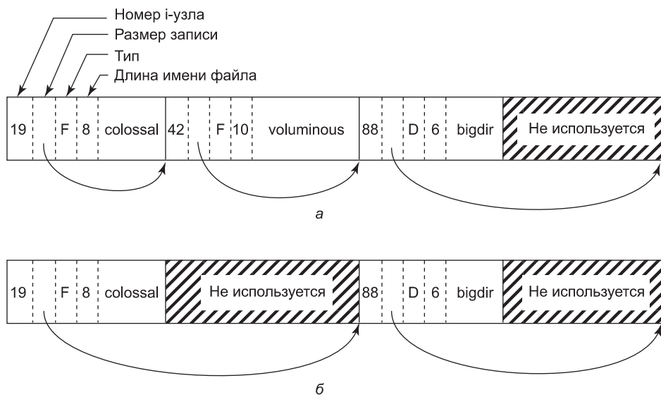
Рис. 10.18. Каталог Linux: a — с тремя файлами; б — после удаления файла voluminous
